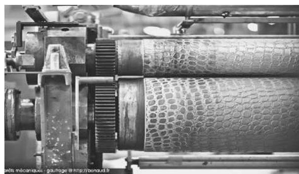
Cylindres de gaufrage
